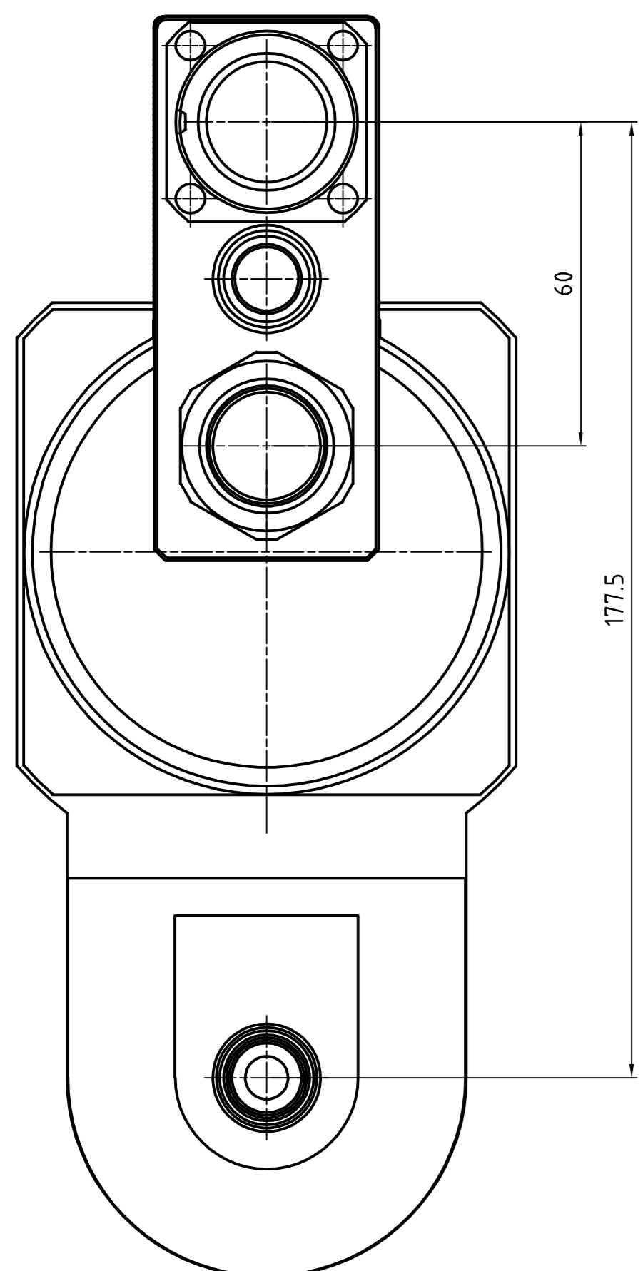
Ansicht "A"
