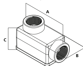
C2 - 2 way 90°
